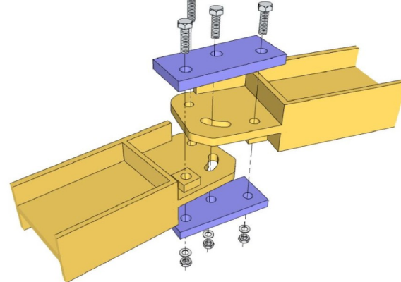
図-4 締結方法
