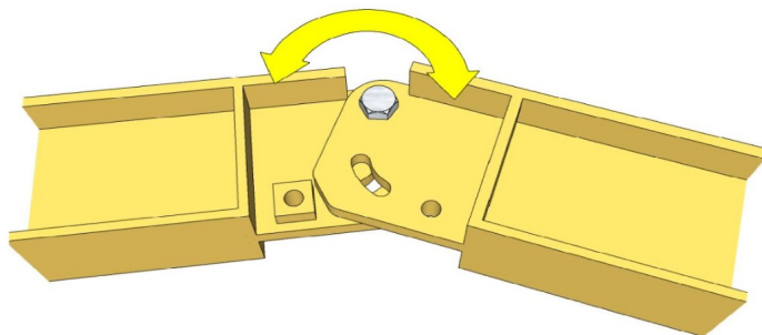
図-7 手順3(角度調整)
