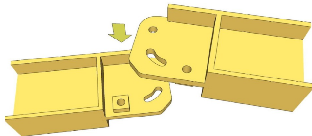
図-5 手順1(基本部材を重ねる)
