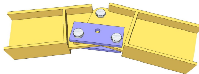
図-8 手順4(プレートをボルトで固定)
